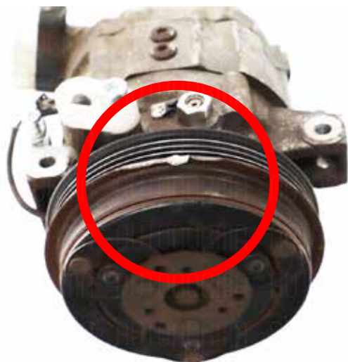
Poškození řemenice kompresoru
